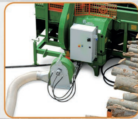
• OPTIONAL ASPIRATORE ELETTRICO PER SEGATURA
